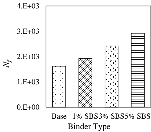
e) Fatigue life, N_f
