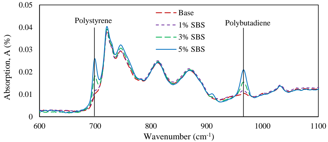
a) FTIR Spectrum
